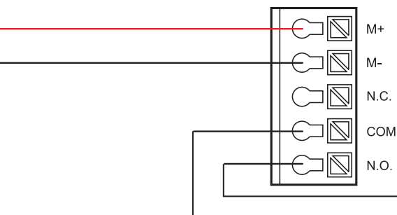
Combiné extérieur
