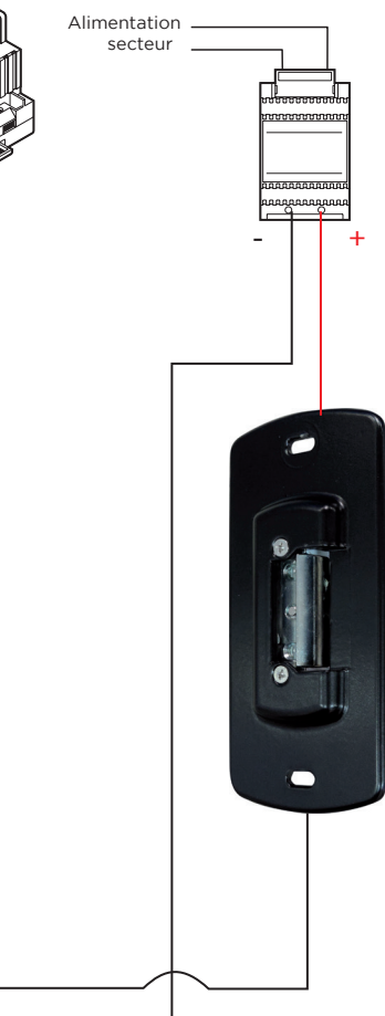
Transformateur 12 V
