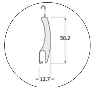
Coupe de la lame
